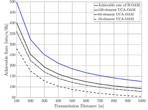
그림 2. H-OAM 시스템의 달성 가능한 속도 성능.
