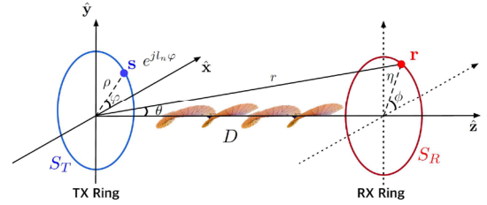
그림 1. 제안하는 연속 링 기반 H-OAM 시스템 모델.
